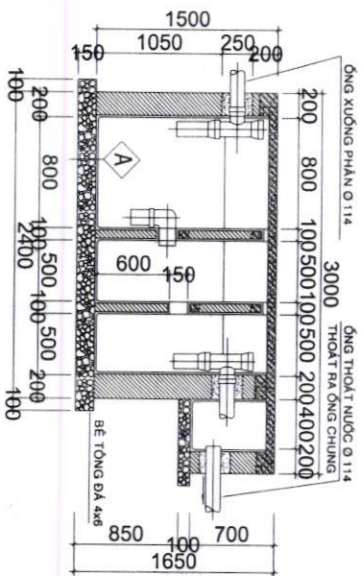
MẶT CẮT A-A BỂ TỰ HOÀI TL:1/50
