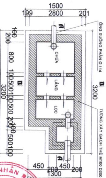
MẶT BẰNG BỂ TỰ HOÀI TL:1/50
