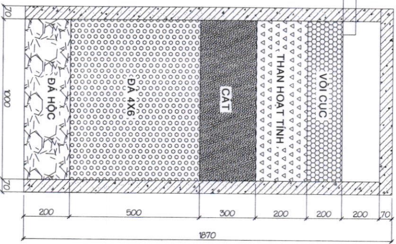
MẶT CẮT GIẾNG THÂM
