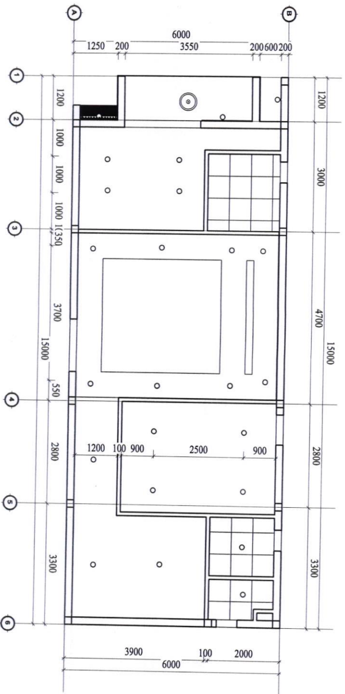
MẶT BẰNG BỐ TRÍ ĐIỆN LẬU 1 TL: 1/100
