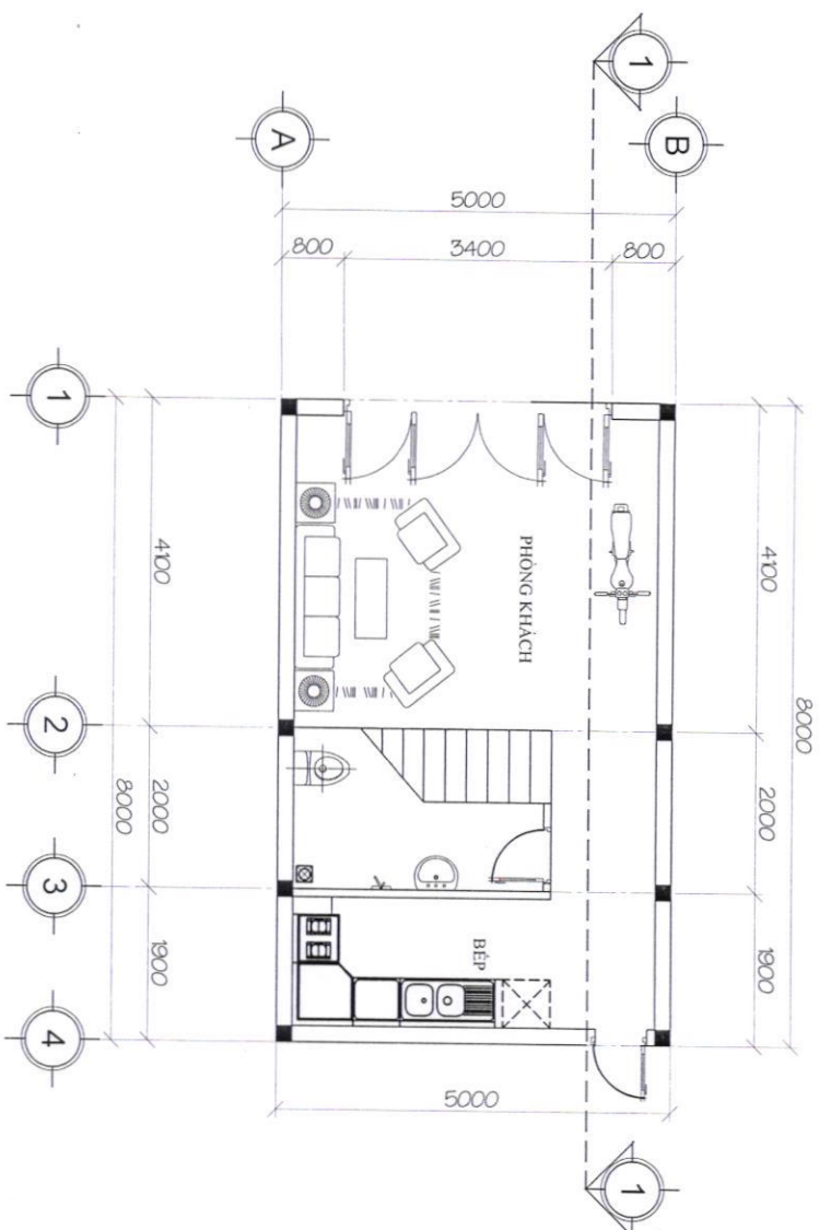
MẶT BẰNG TẦNG TRỆT TL 1:100
