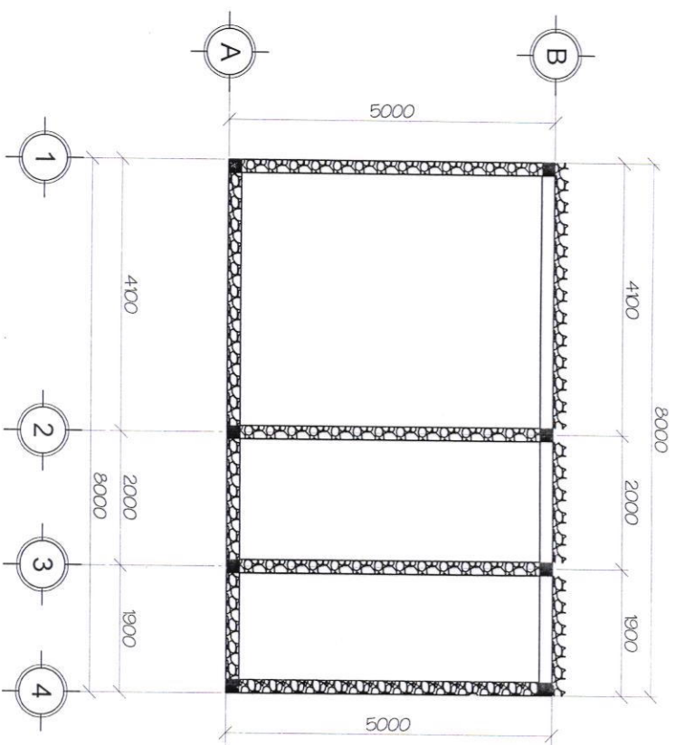
MẶT BẰNG DÀ KIỀNG TL 1:100
