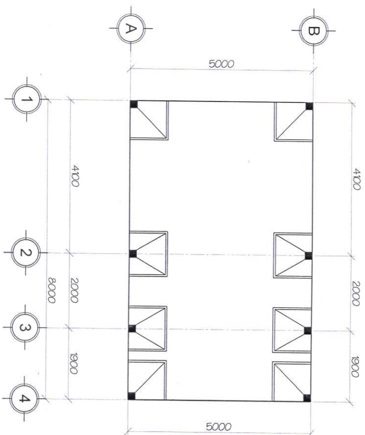
MẶT BẰNG MÓNG TL 1:100
