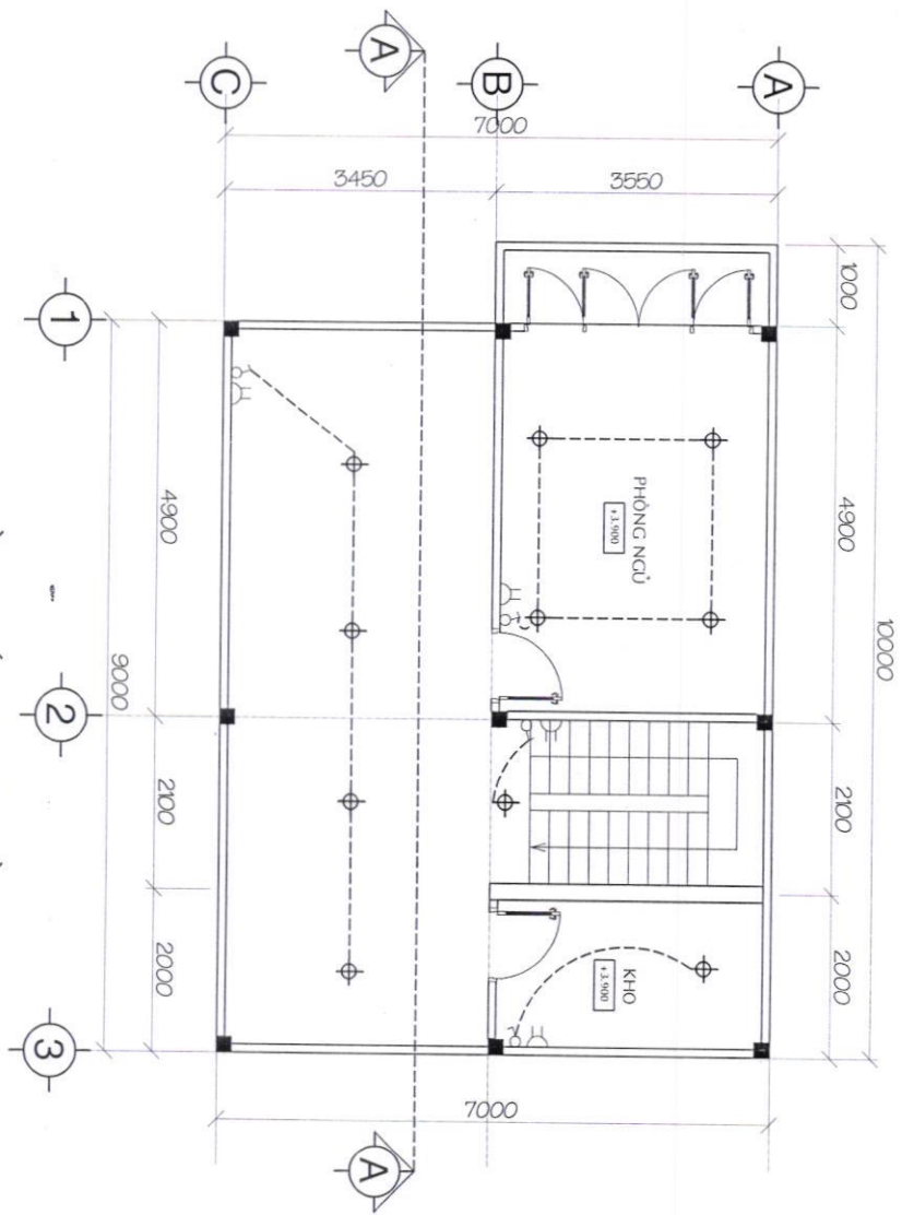
MẶT BẰNG BỐ TRÍ ĐIỆN LẦU 2 TL 1/100
