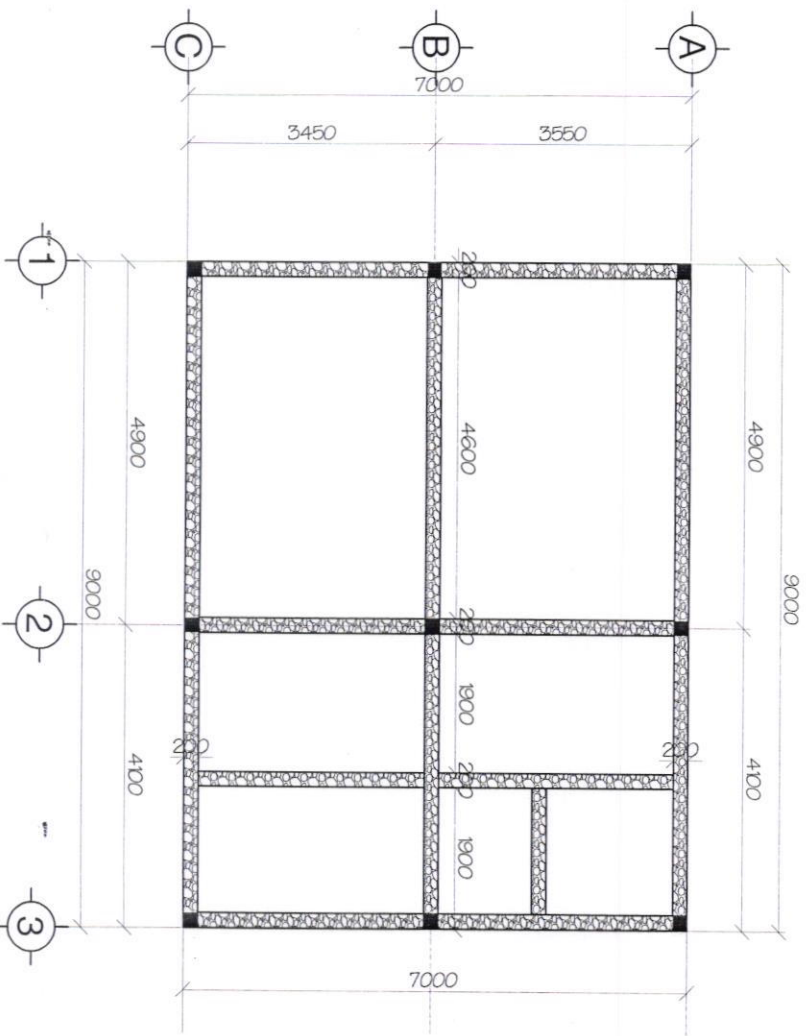
MẶT BẰNG DÀ KIẾN TL 1/100
