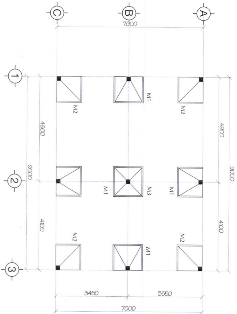
MẶT BẰNG BỐ TRÍ MỘNG TL 1/100
