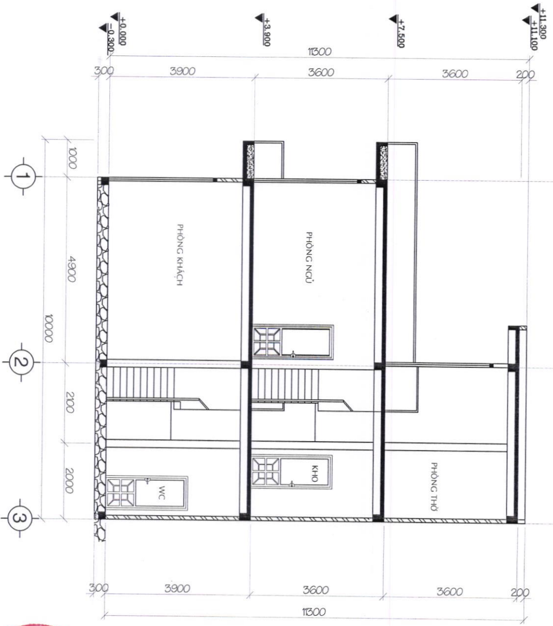
MẶT CẮT A-A TL 1/100
