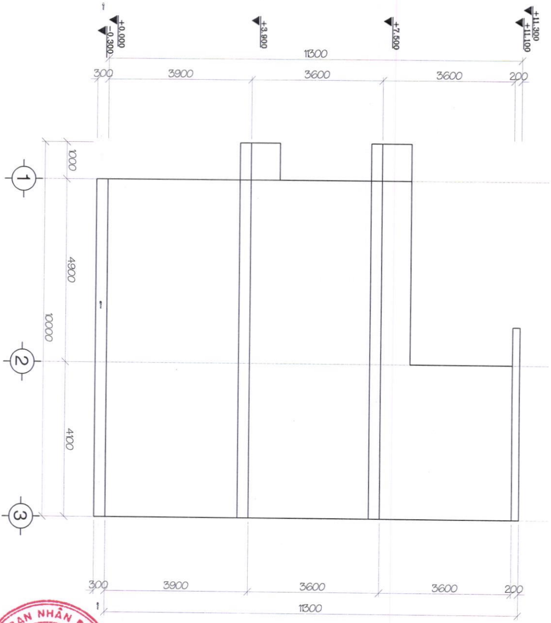
MẶT ĐỨNG TRỤC 1-4 TL 1/100
