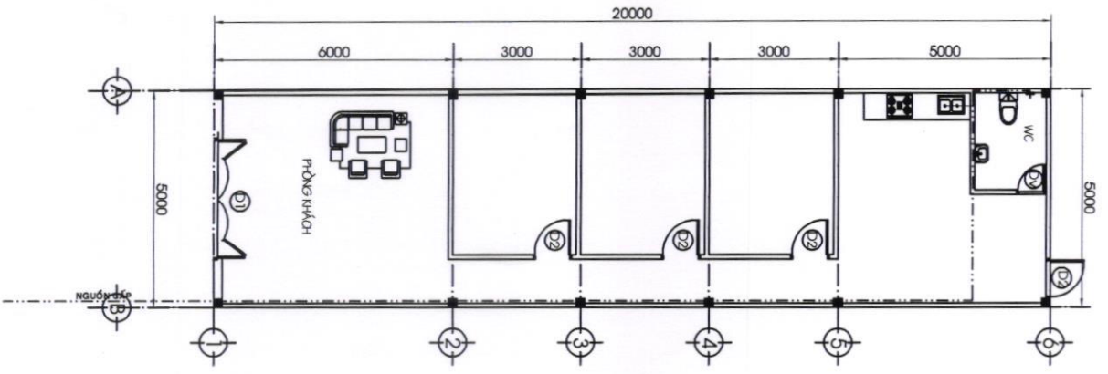
MẶT BẰNG CẤP NƯỚC TL 1/100
