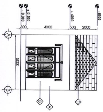
MẶT ĐỪNG CHÍNH TL 1/100
