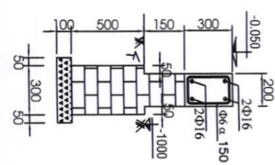
MD-1: TL:1/20
