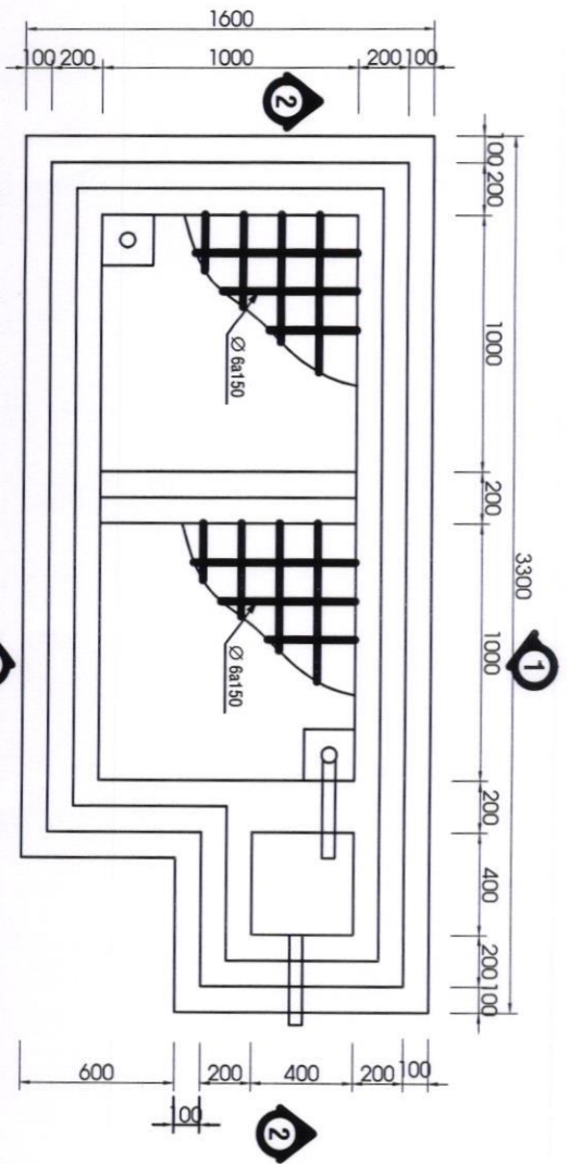
MBÀNG HẦM TỰ HOẠI : TL 1/20
