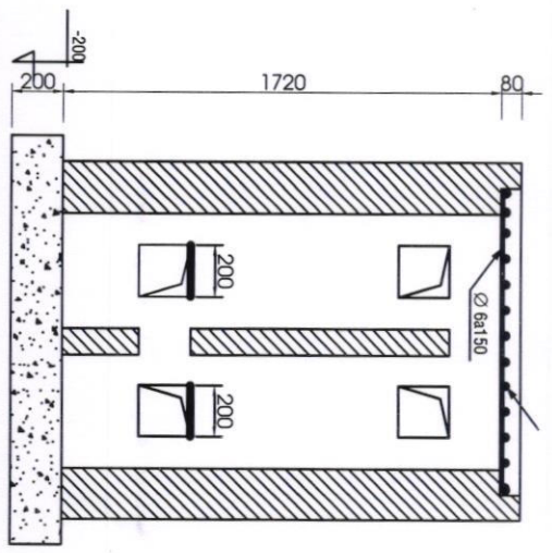
M.CẮT 1-1 : TL 1/20
