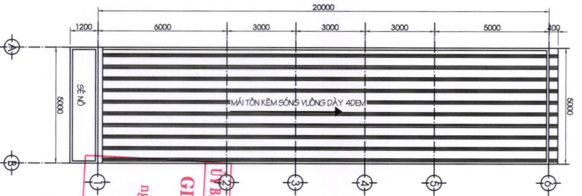
MẶT BẰNG MÁI TL 1/100
