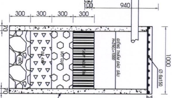
M.CẮT 3-3 : TL 1/20
