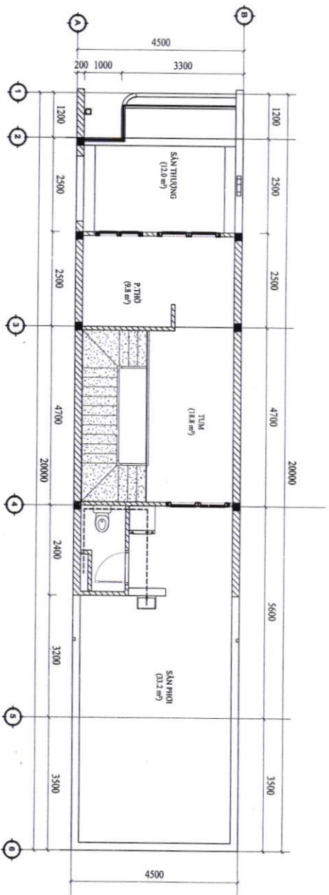
MẶT BẰNG CẤP NƯỚC TẦNG 3 TL 1/100
