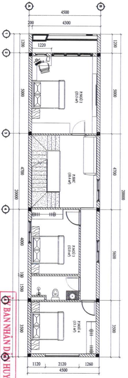
MẶT BẰNG TẦNG 2 TL 1/100
