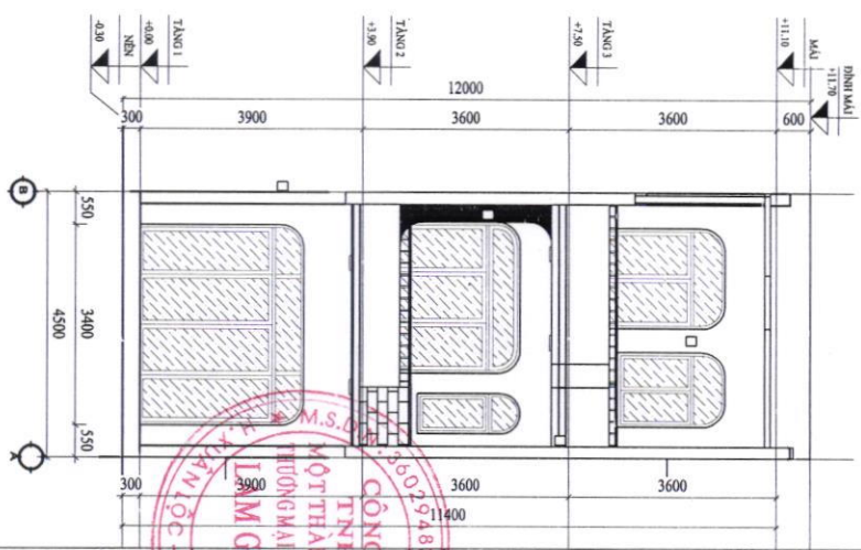
MẶT ĐỨNG TRỰC A-B TL 1/100
