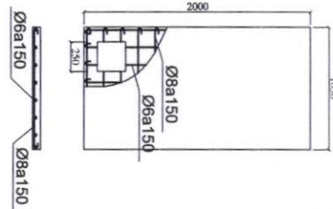
DÀN HẦM CHỨA
