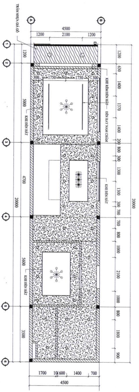
MẶT BẰNG ĐÈN TRẦN TẦNG TRỆT TL 1/100
