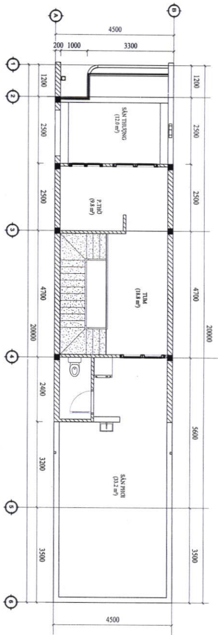
MẶT BẰNG TẦNG 3 TL 1/100
