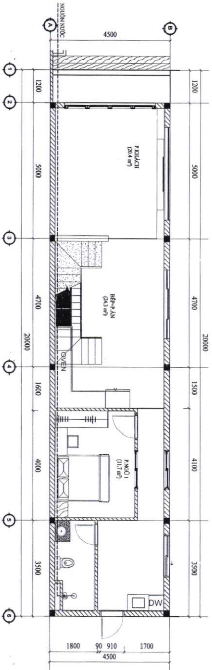
MẶT BẰNG CẤP NƯỚC TẦNG TRỆT TL 1/100
