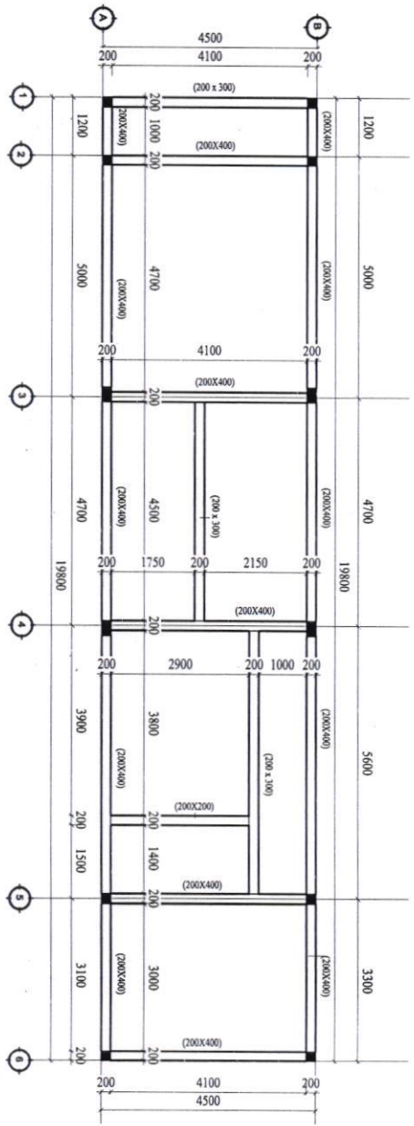
MẶT BẰNG DÀ KIỀNG TẦNG 2 TL 1/100
