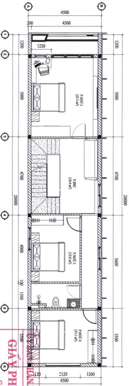
MẶT BẰNG CẤP NƯỚC TẦNG 2 TL 1/100
