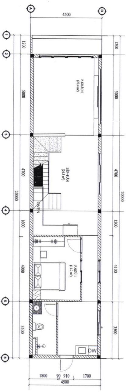
MẶT BẰNG TẦNG TRỆT TL 1/100
