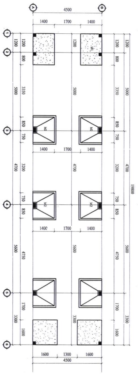
MẶT BẰNG MÔNG TL 1/100
