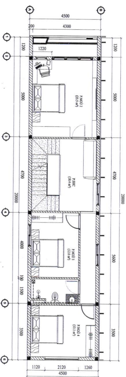
MẶT BẰNG THOÁT NƯỚC TẦNG 2 TL 1/100
