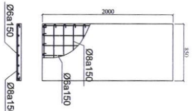
DÀN HẦM LỌC
