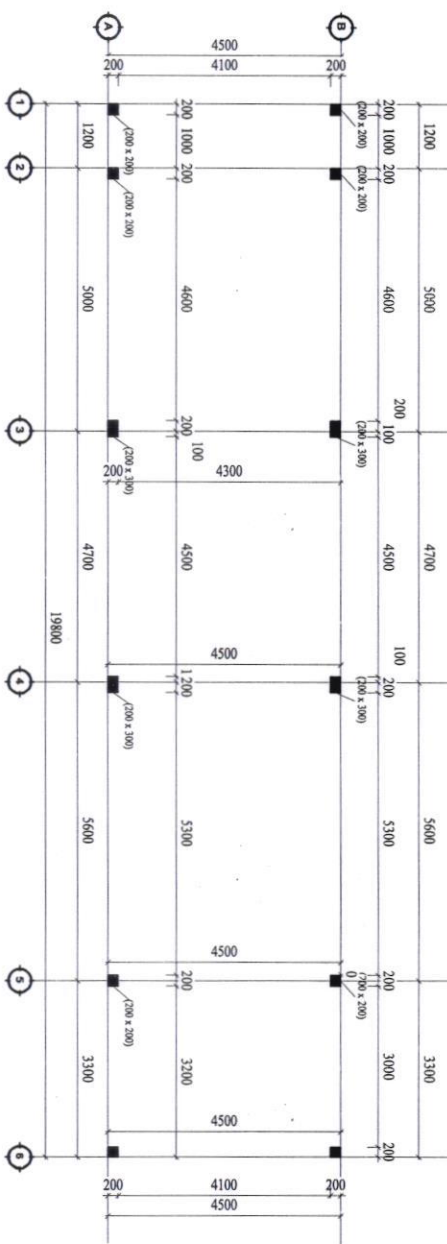
MẶT BẰNG CỘT TL 1/100
