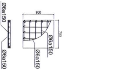
DÀN HẦM HG
