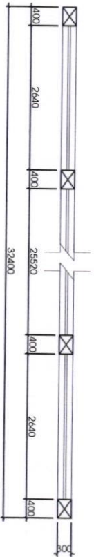
MẶT BẰNG HÀNG RÀO ĐOẠN XÂY MỚI 5-A TL: 1/50
