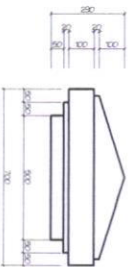
CHI TIẾT A TL:1/10
