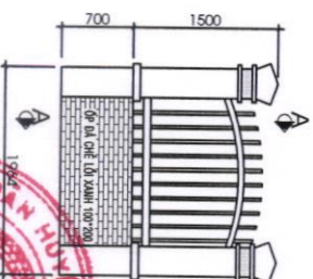
MẶT ĐƯỜNG HÀNG RÀO XÂY MỚI 4-5 TL : 1/50
