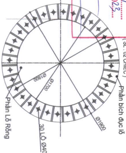
BÍCH ĐỊNH VỊ BULÔNG - DÂY 10mm ( SL : 02 CHIẾC )
