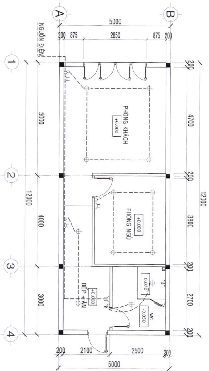
MẶT BẰNG CẤP ĐIỆN TL 1:100
