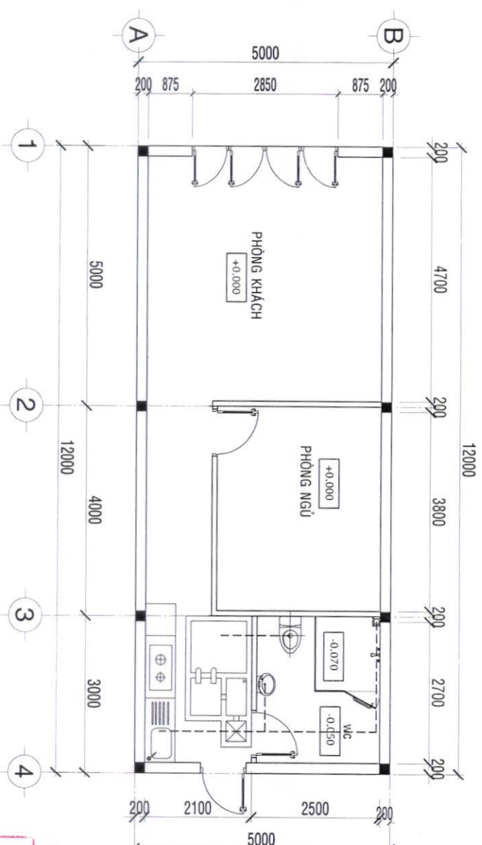
MẶT BẰNG THOÁT NƯỚC TL 1:100
