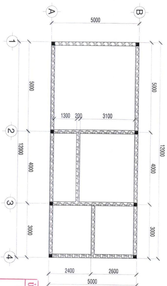
MẶT BẰNG DÀ KIỂNG TL 1:100
