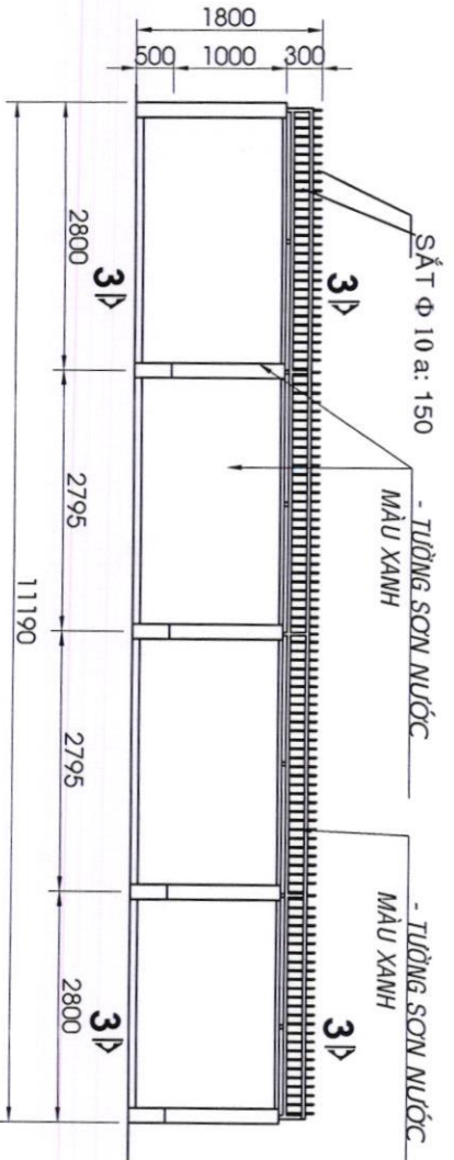
- TƯỜNG RÀO ĐOẠN D - 3 CHIỀU DÀI 11,19 M
